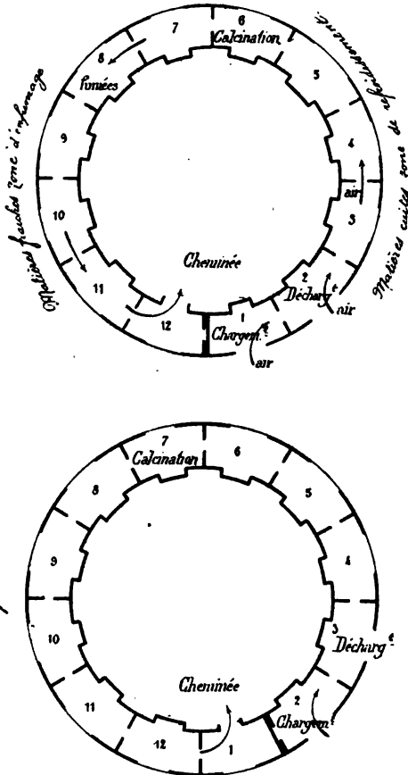
Fig. 70, 74. — Fours-annulaires.
